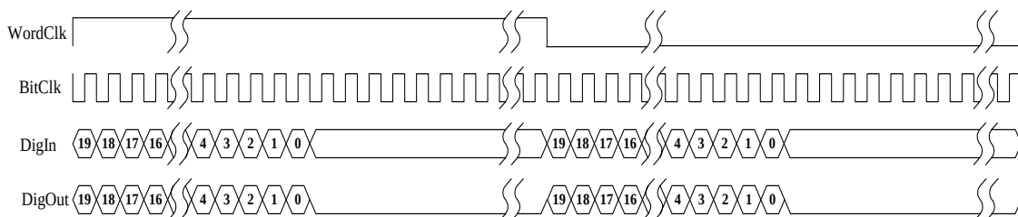
图. DigIn/DigOut 时序图
