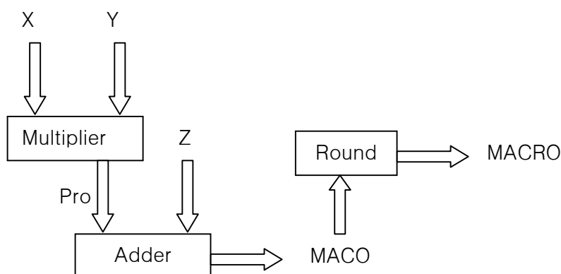
MAC 构架图
