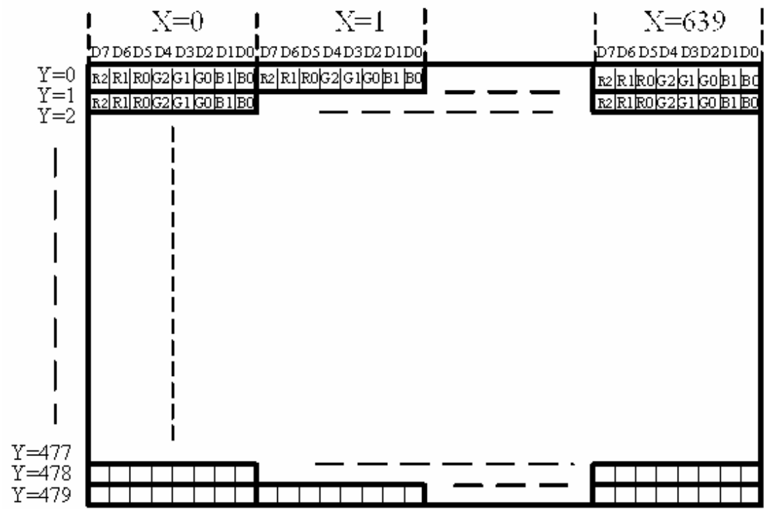
图 2 显示存储器与像素对应关系
