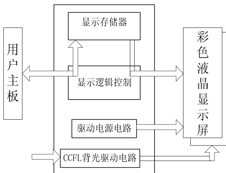
图 1 TFT3224-5.7 原理框图
