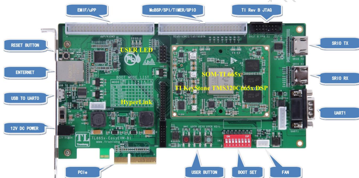
图 10 硬件资源图解
