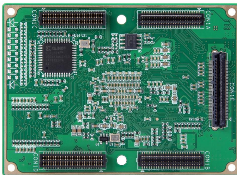
图 7 SOM-TL665x 背面
