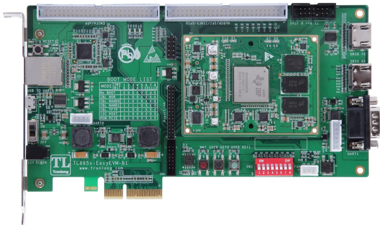
图 1 TL665x-EasyEVM 正面
