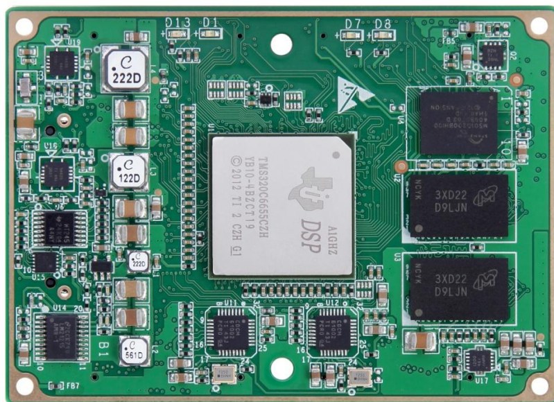
图 6 SOM-TL665x 正面
