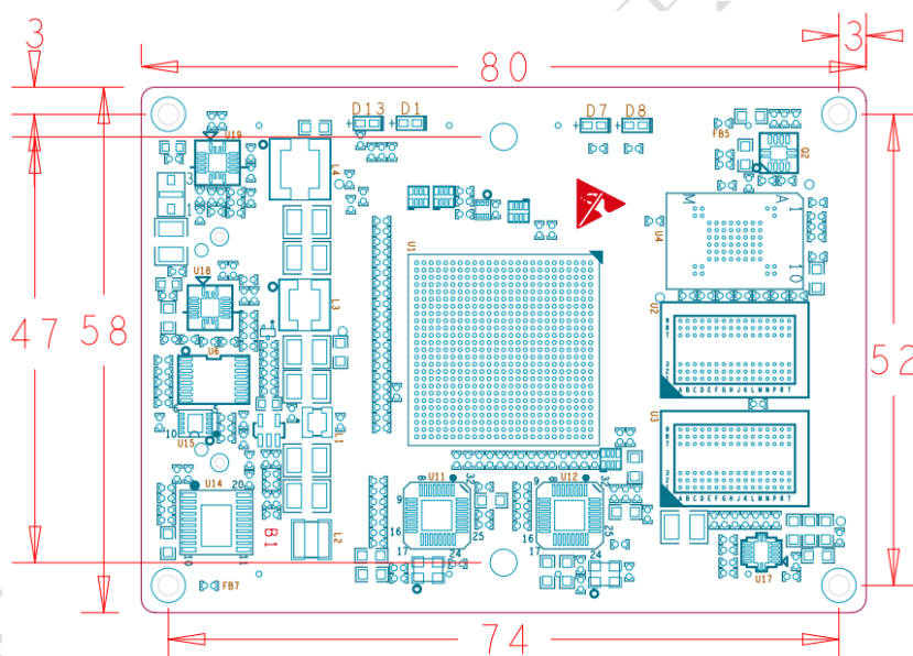
图 14 SOM-TL665x 机械尺寸图
