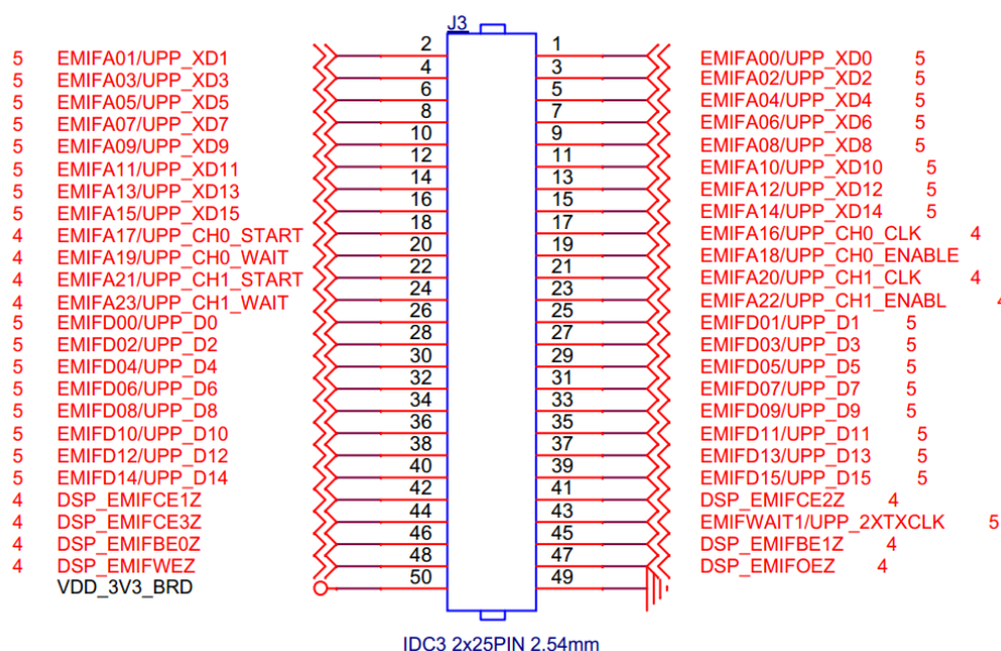
图 12 J3 连接器：uPP、EMIF 等拓展信号定义
