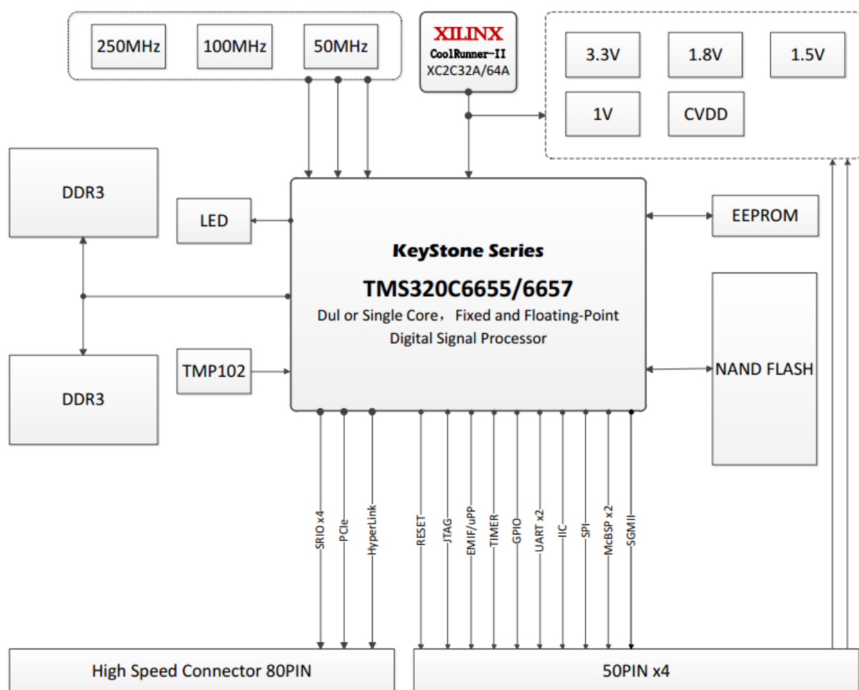
图 8 SOM-TL665x 硬件框图
