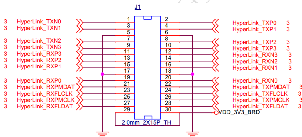
图 11 J1 连接器：HyperLink 拓展信号定义
