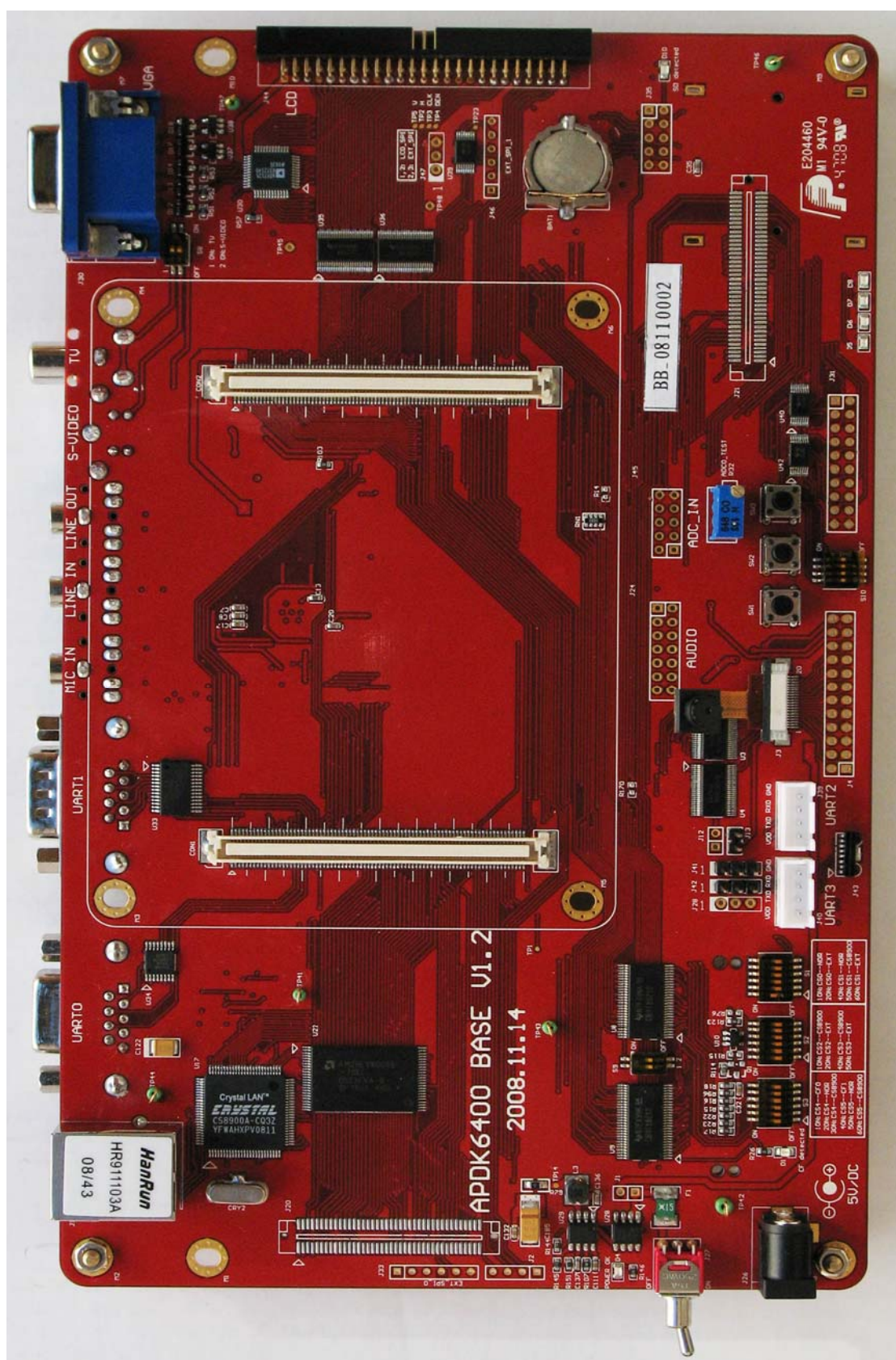
图 3-2 底板实物图
