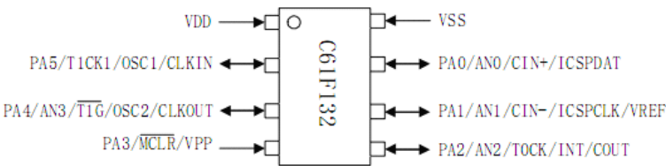
DIP/SOIC/TSSOP 管脚图
