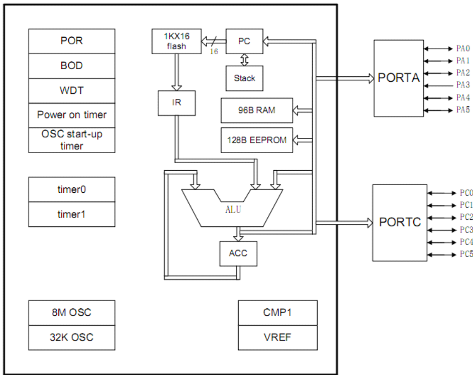
模块框图
