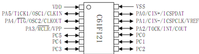
DIP/SOIC/TSSOP 管脚图
