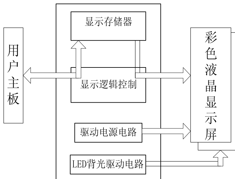
图 1 TFT3224-3.5 原理框图
