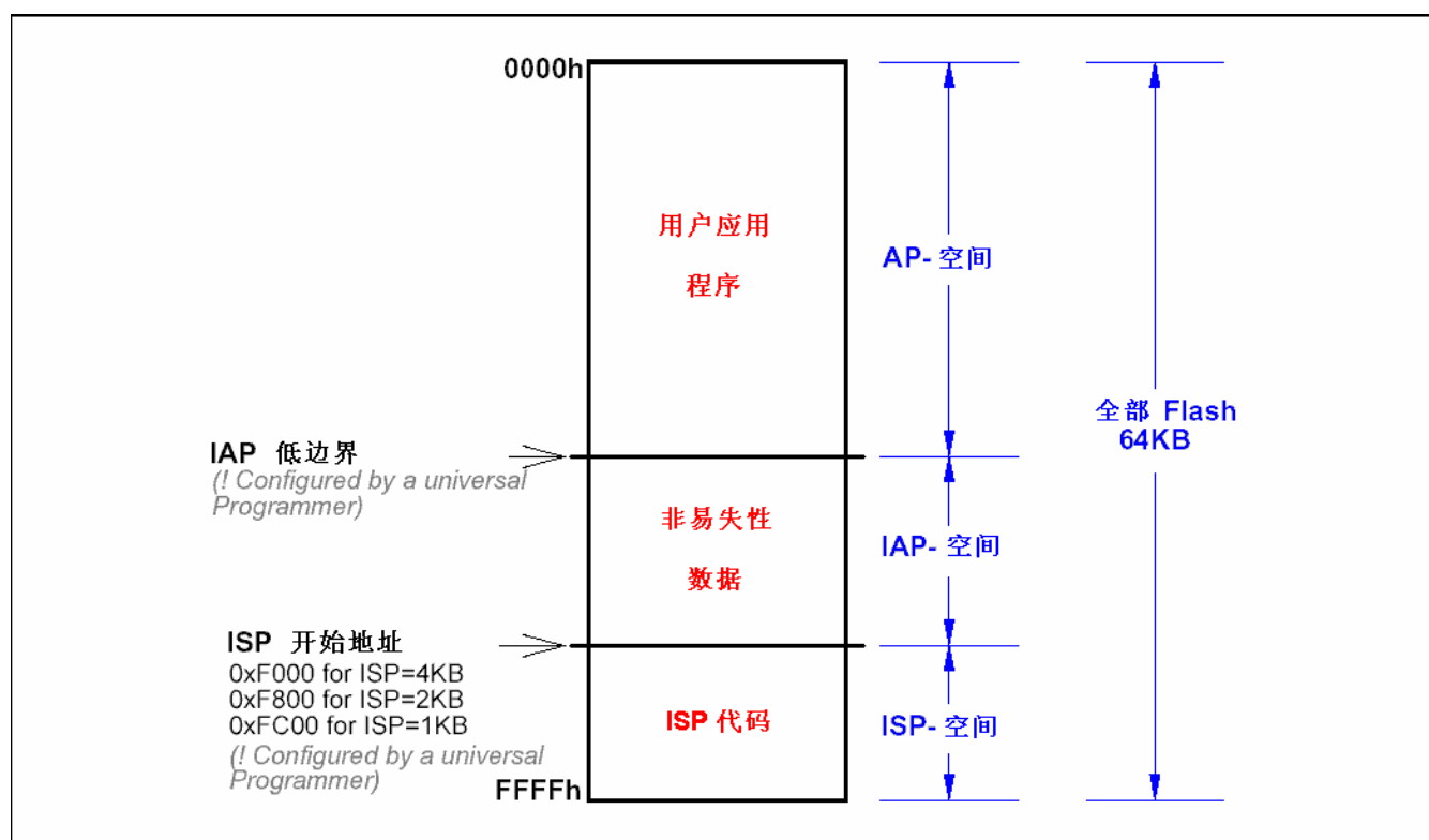
图 20-1. Flash 结构
