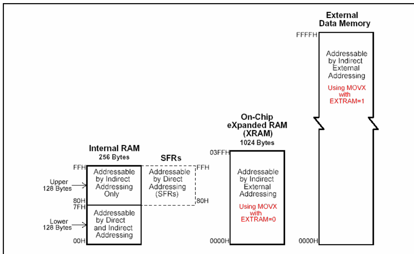
Figure 5-2. 数据存储器
