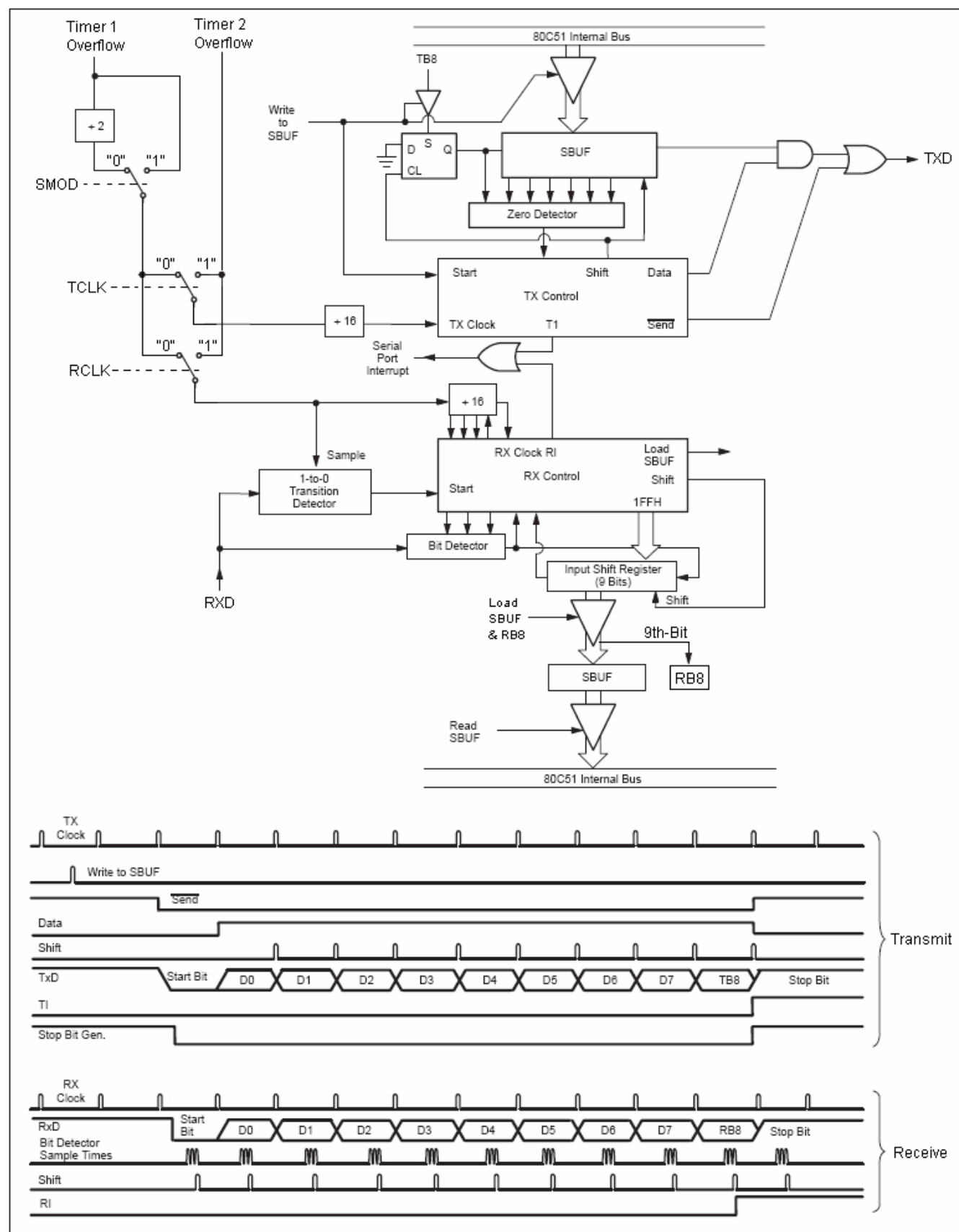
图 12-4 串行口模式 3
