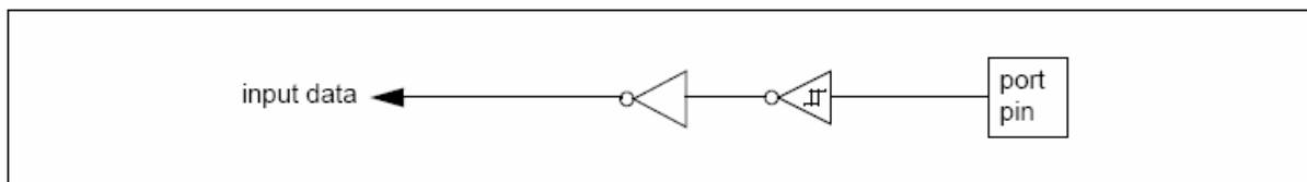
图 10-3 输入
