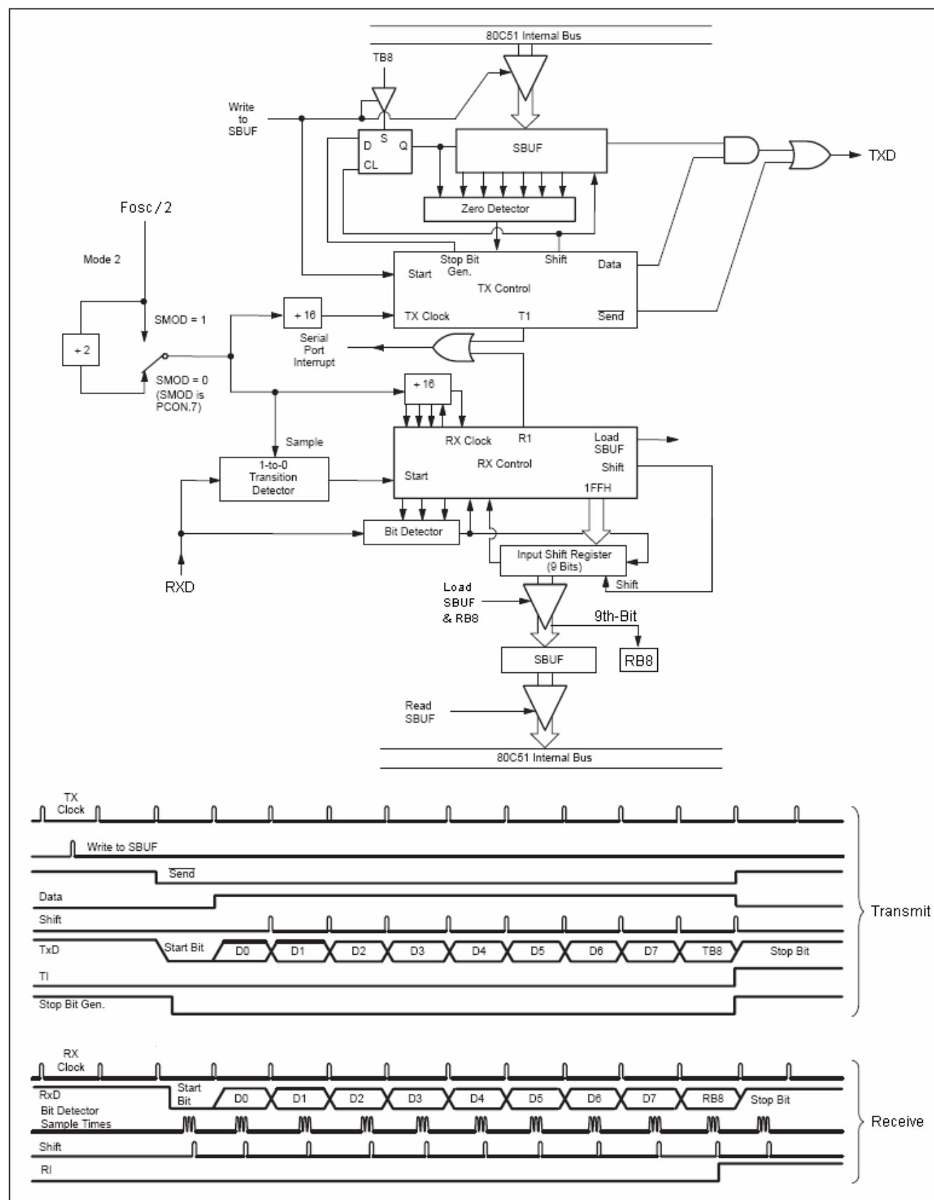
图 12-3 串行口模式 2
