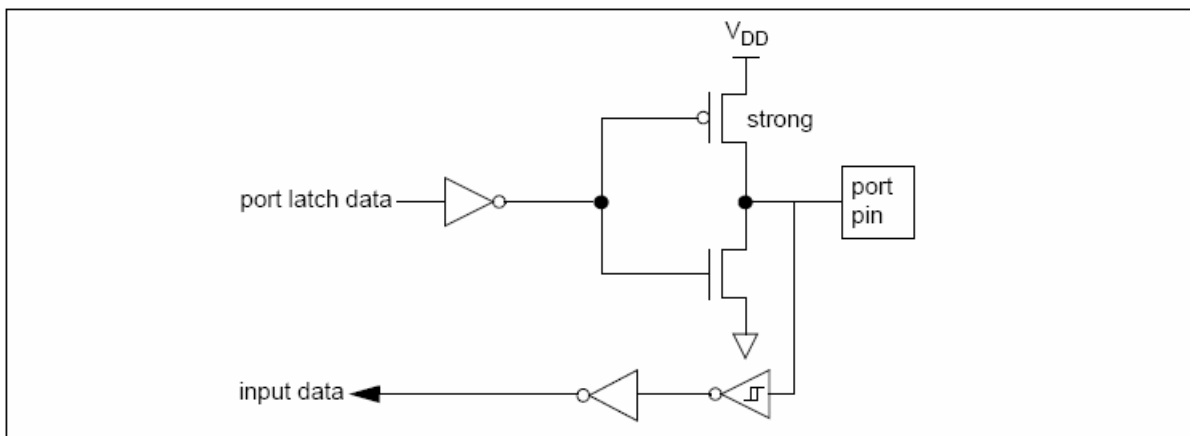
图 10-4 上拉输出
