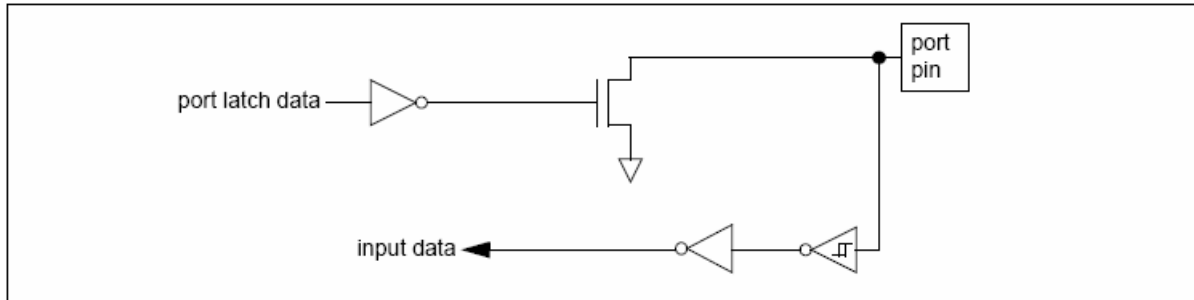
图 10-2 开漏输出
