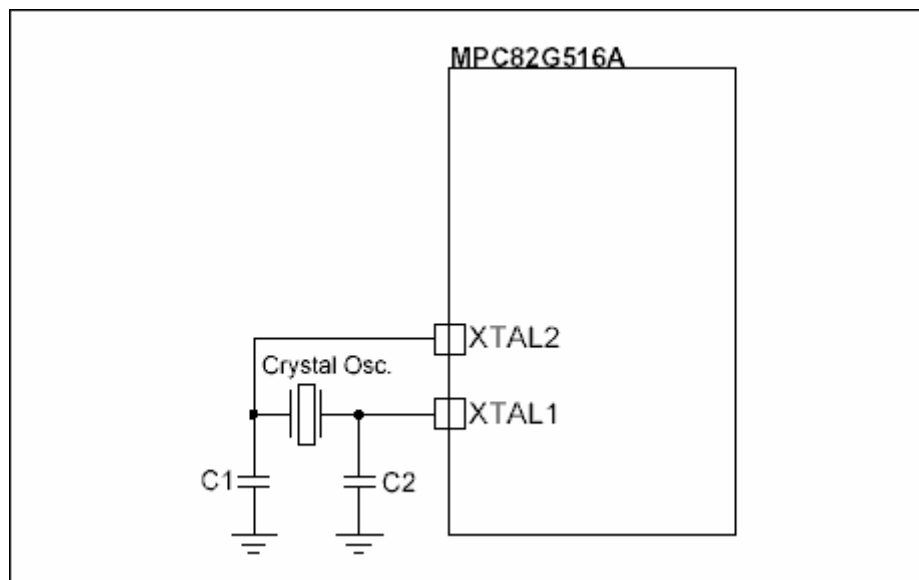
图 27-5. 晶振电路
