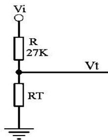
图 4 热敏电阻应用电路图
