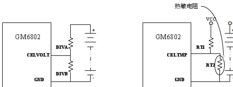
图 2 电池电压和温度检测原理图
